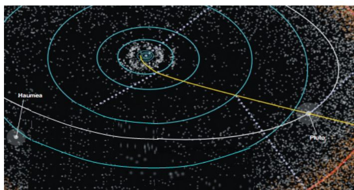
Hình 1: quỹ đạo của con tàu New Horizons từ Trái đất đến biên giới của thái dương hệ. New Horizons sẽ tiếp cận Pluto và PT1
