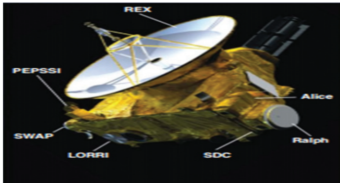
Hình 5: các thiết bị hiện đại trên New Horizons
