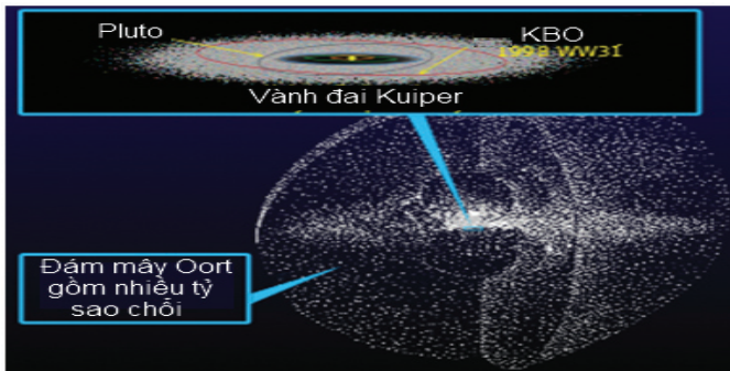
Hình 3: đám mây Oort và vành đai Kuiper với Pluto và KBO 1998 WW31
